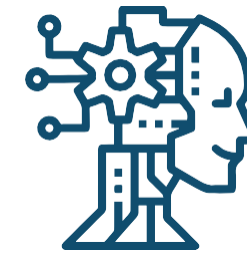
AI & ML
